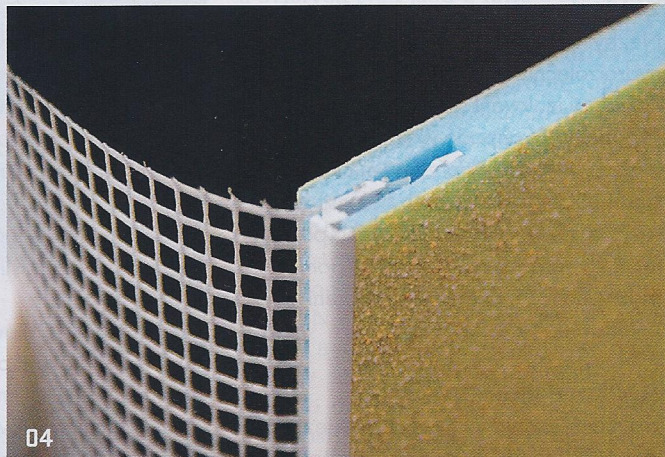
04 > Prefabrikované ostění - rovná deska (detail)
