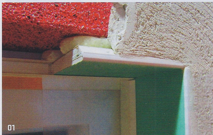
01 > Varianta prefabrikovaného ostění pro vnitřní stavbu (sádrokarton)
